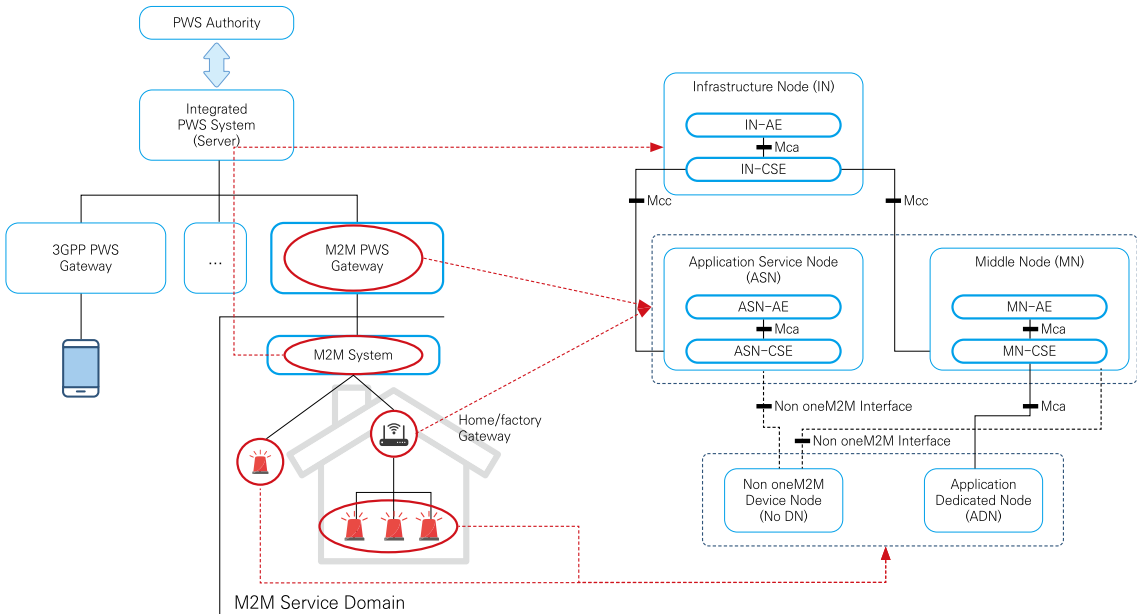
[그림 8] oneM2M 기반 공공안전 알람 서비스 참조구조
