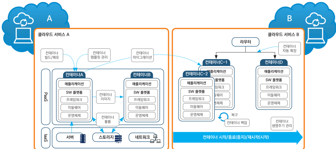
[그림 3] PaaS 상호운용성 시험 구성도 예시
